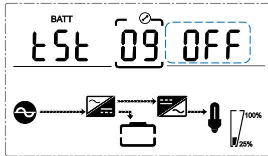
Fig. 4-21 Ajuste del autotest de la batería
