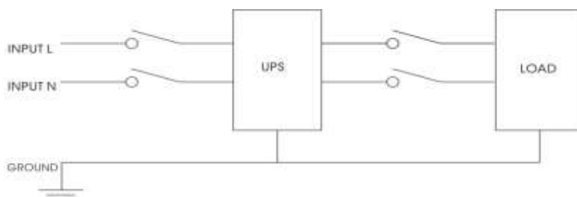
Fig. 3-1 Configuración correcta
