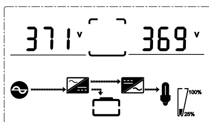
Fig. 4-11 Tensión del bus DC interno
