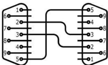
Fig. 5-3 Conexión PC a SAI
