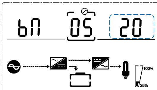
Fig. 4-17 Ajuste de la cantidad de baterías
