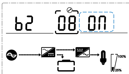
Fig. 4-20 Ajuste del indicador acústico
