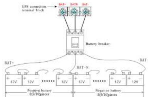
Fig. 3-4 Conexión de baterías externas
