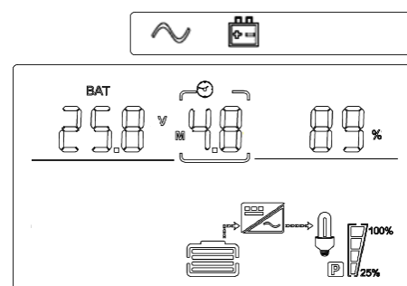
Fig. 4-3 Panel de control en modo batería
