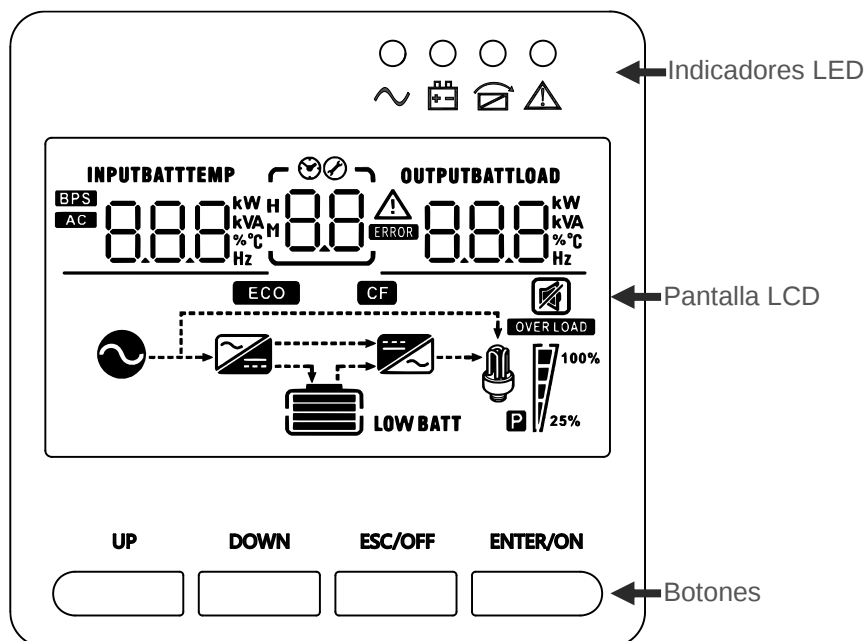
Fig. 4-1 Panel de control del SAI
