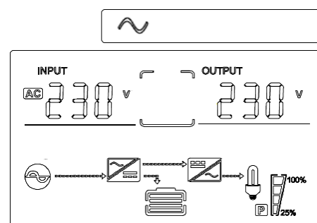
Fig. 4-2 Panel de control en modo Online
