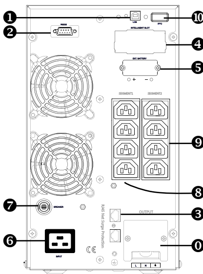
ZGR TOWER PRO 2KVA ZGR TOWER PRO 2KVA LBT
