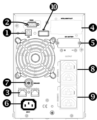
ZGR TOWER PRO 1KVA ZGR TOWER PRO 1KVA LBT
