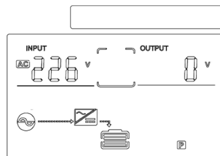
Fig. 4-5 Panel de control en modo standby
