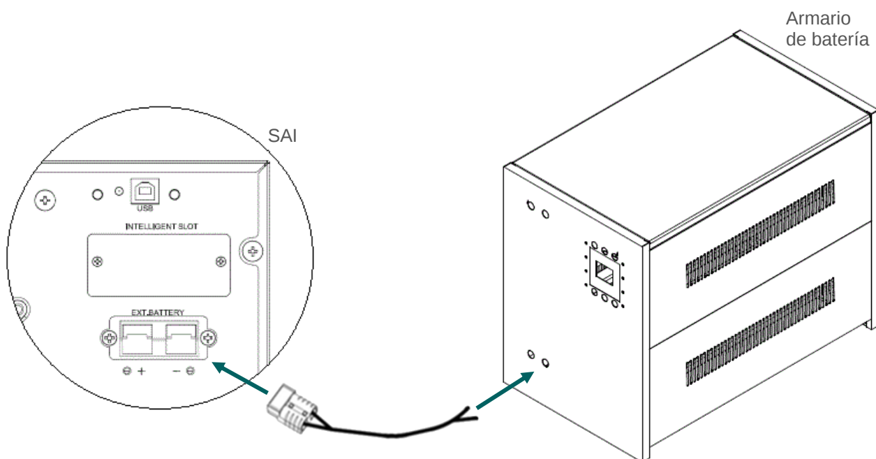
Fig. 3-3 Imagen ilustrativa de conexionado de batería con armarios de la serie "A"
