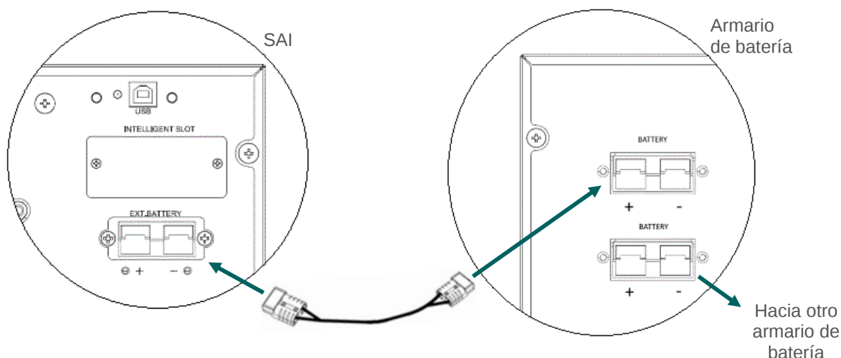
Fig. 3-2 Imagen ilustrativa de conexionado de batería con armarios tipo TOWER PRO
