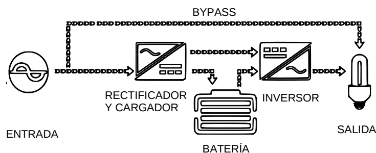
Fig. 2-1 Diagrama de bloques del SAI ZGR TOWER PRO 1 – 3 KVA
