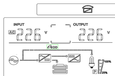
Fig. 4-6 Panel de control en modo ECO
