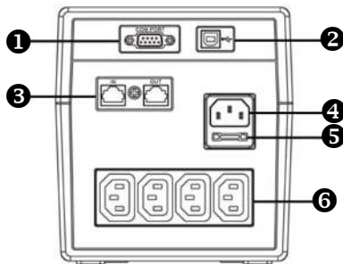
Trasera de ZGR STEADY 1000
